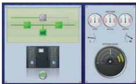
Diagrama de estado, mediciones y unifilar del sistema.
